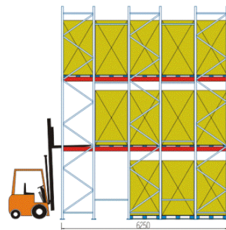
驶入式货架 侧视图
