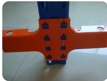
牛腿结构 (SuPPORT)
