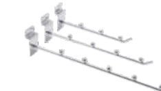
E017 Slatwall hook 万用板 直5, 6, 7, 8, 9珠 Thickness(厚度): \phi 8\text{ mm} , \phi 10\text{ mm} . Length (长度): 200, 250, 300, 350mm
