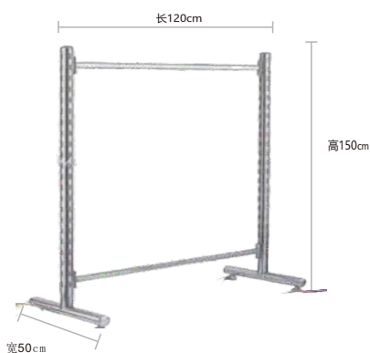
YG-S20 50圆管长方双孔
