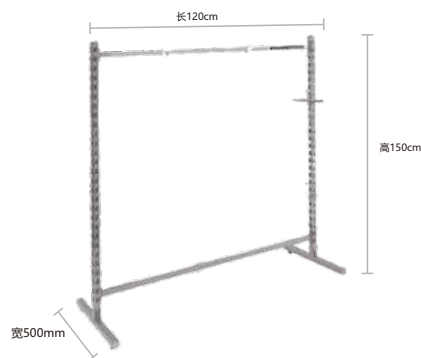
YG-S21 38方管长方双孔
